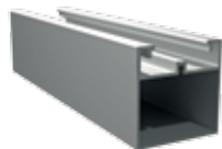
Hliníkový profil pro samonosné konstrukce nebo připevnění k podkladu (podpěrné body každých 70 cm) 50 × 50 mm
